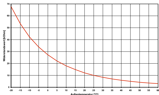
Abb. 7.2: Fühlerkennlinie NTC-10
